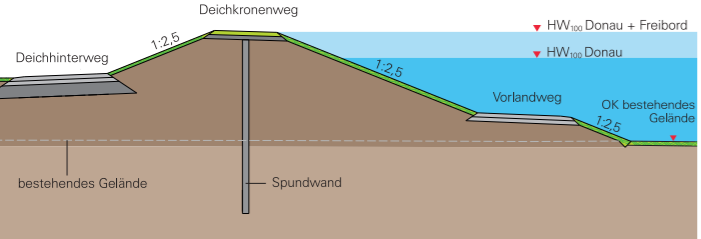
▲ Polder 1 - Regelquerschnitt Deichneubau
