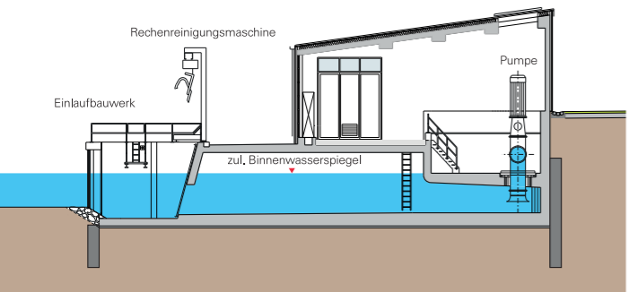
▲ Polder 1 - Schöpfwerk Winzer 1 mit Einlaufbauwerk - Neubau
