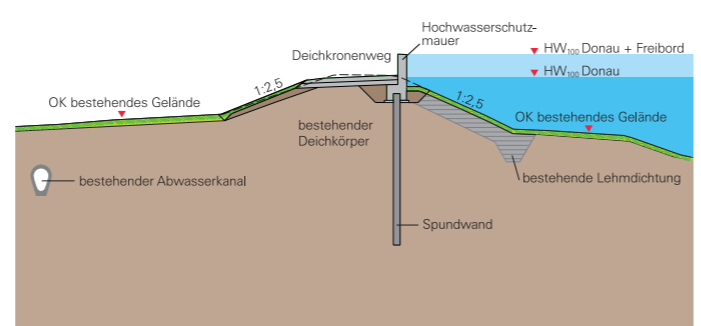
▲ Polder 2 - Regelquerschnitt Deichaufhöhung mit HWS-Mauer
