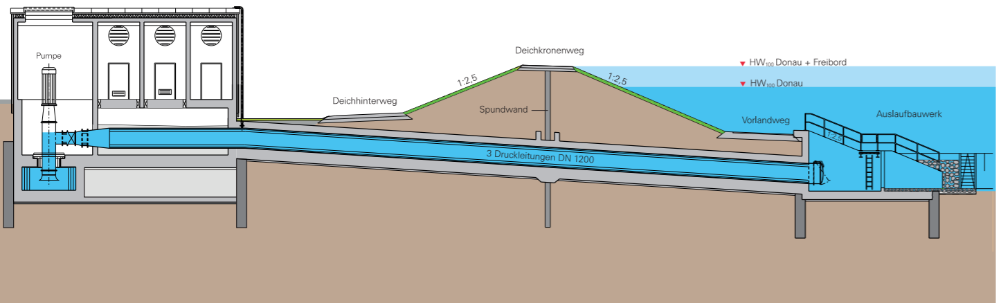
▲ Polder 1 - Schöpfwerk Winzer 1 mit Deich- und Auslaufbereich - Neubau
