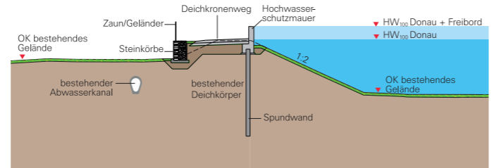
▲ Polder 1 - Regelquerschnitt Deichaufhöhung mit HWS-Mauer
